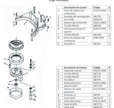
Figura N°7: Set de soporte del contenedor, soporte planetario y eje mezclador
