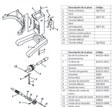
Figura N°4: Set de elevación de la rueda lateral, posterior y trasera
