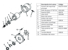
Figura N°4: Set de motor
