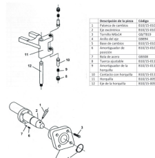
Figura N°5: Set de horquilla y eje de desplazamiento
