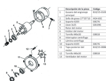
Figura N°4: Set del motor
