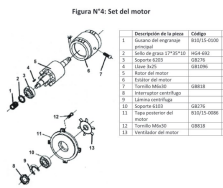
Figura N°4: Set del motor
