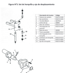
Figura N°5: Set de horquilla y eje de desplazamiento
